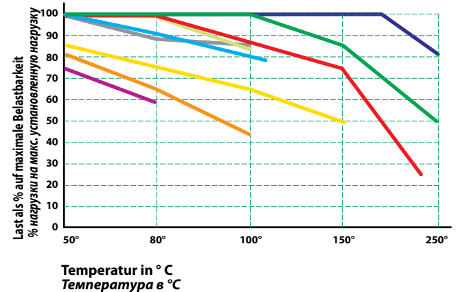
Belastbarkeit/Temperatur Мощность/Температура
