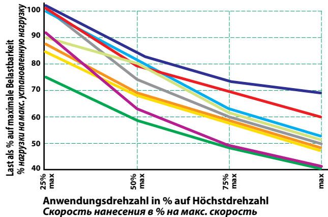
Belastbarkeit/Geschwindigkeit Мощность/Скорость
